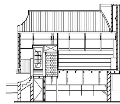
langsdoorsnede
